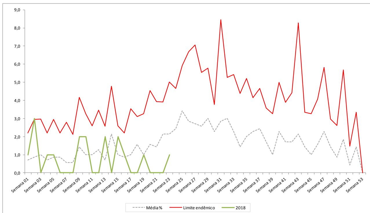
Figura 4 Diagrama de controle do número de casos de Doença Meningocócica, RS, 2000-2017*
